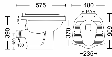
ANGLO-P 8102 575 x 480 x 390mm
